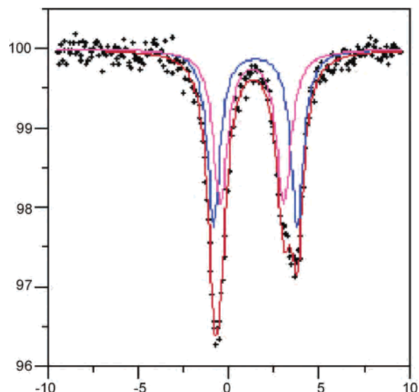
Figure 7. Mössbauer spectrum of [ ^n\text{Bu}_2\text{Sn} (oda)(H _2 O)] _2 ( 2 ).
